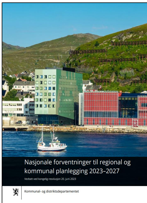
Figur 3. Nasjonale forventningar 2023-27.
